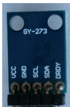
Figura 21. HMC5883L. Part posterior
