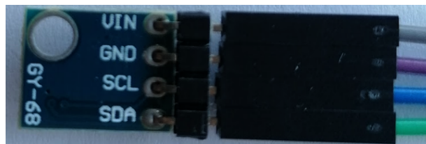
Figura 15. BMP180. Part posterior
