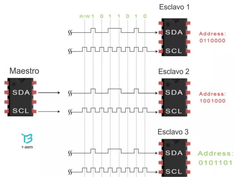
Figura 68. Els esclaus comparen la direcció enviada amb la seva
